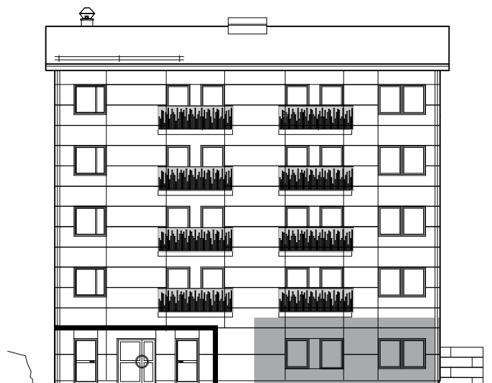
FASAD MOT NORDVÄST
